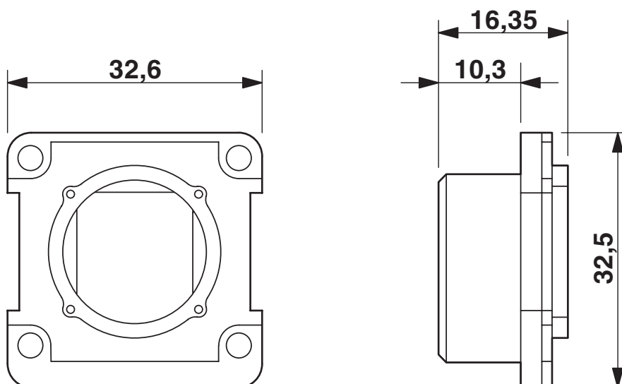
Rysunek wymiarowy
