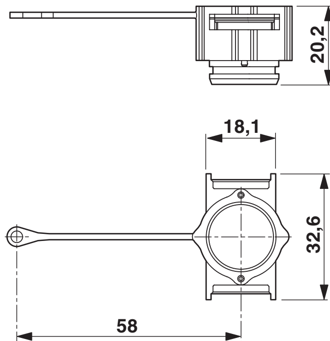
Rysunek wymiarowy
