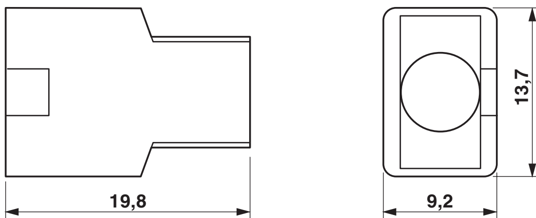
Rysunek wymiarowy
