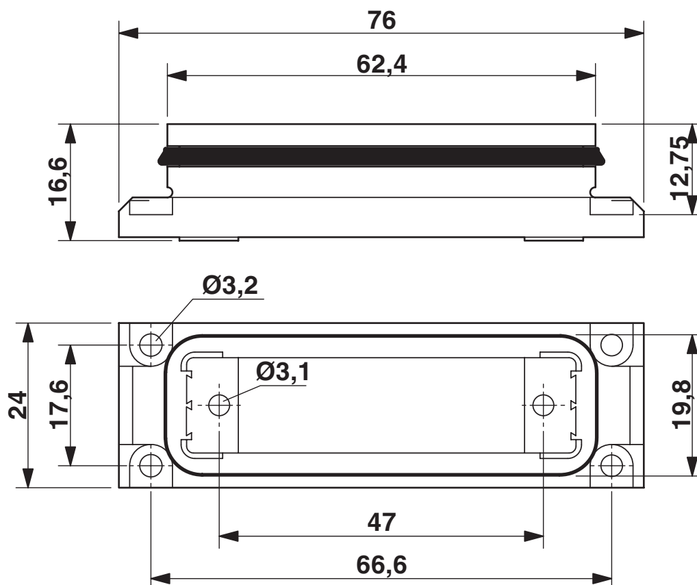
Rysunek wymiarowy
