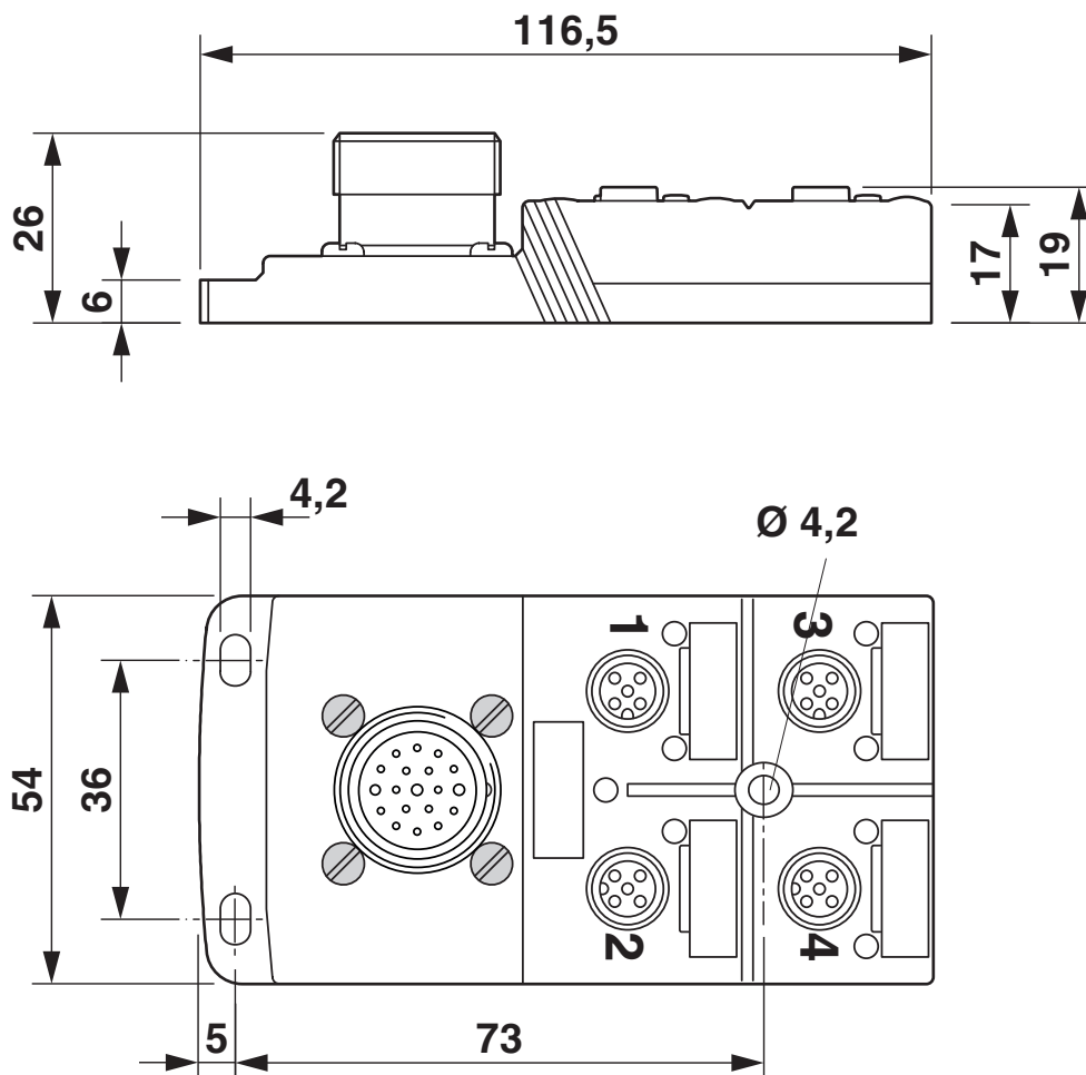
Rysunek wymiarowy
