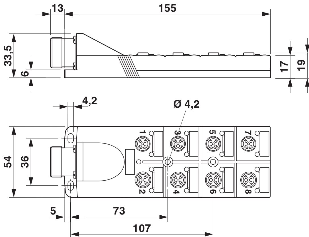
Rysunek wymiarowy
