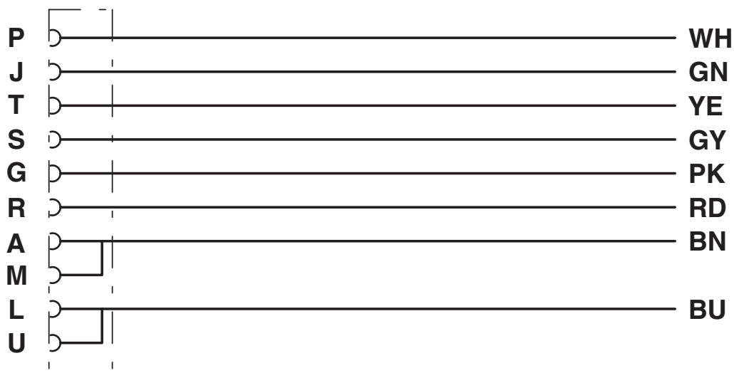
Schemat
