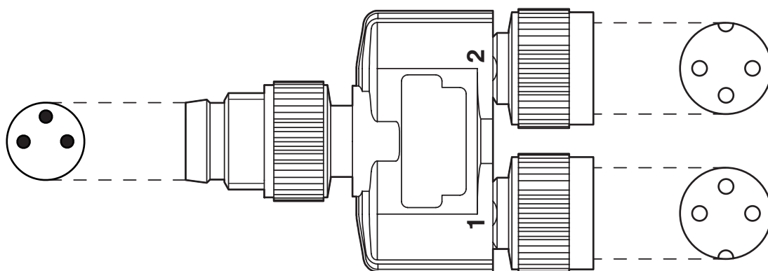
Orientacja układu pinów
