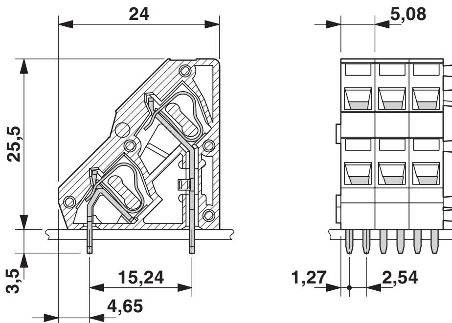
Rysunek wymiarowy
