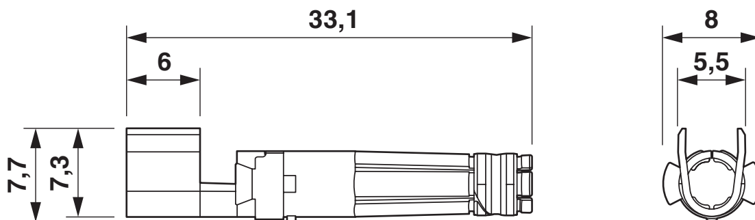
Rysunek wymiarowy
