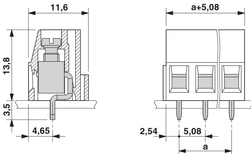
Rysunek wymiarowy
