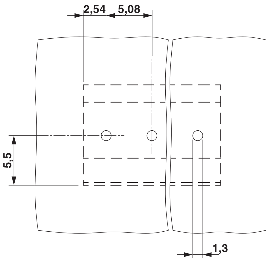
Otworowanie/geometria płytek lutowniczych
