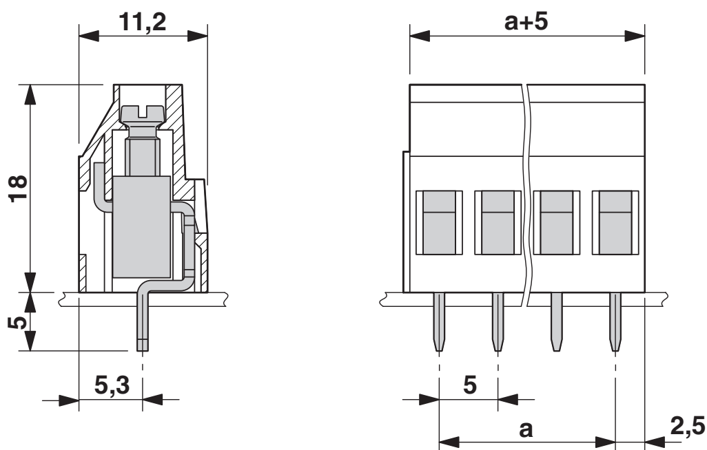
Rysunek wymiarowy
