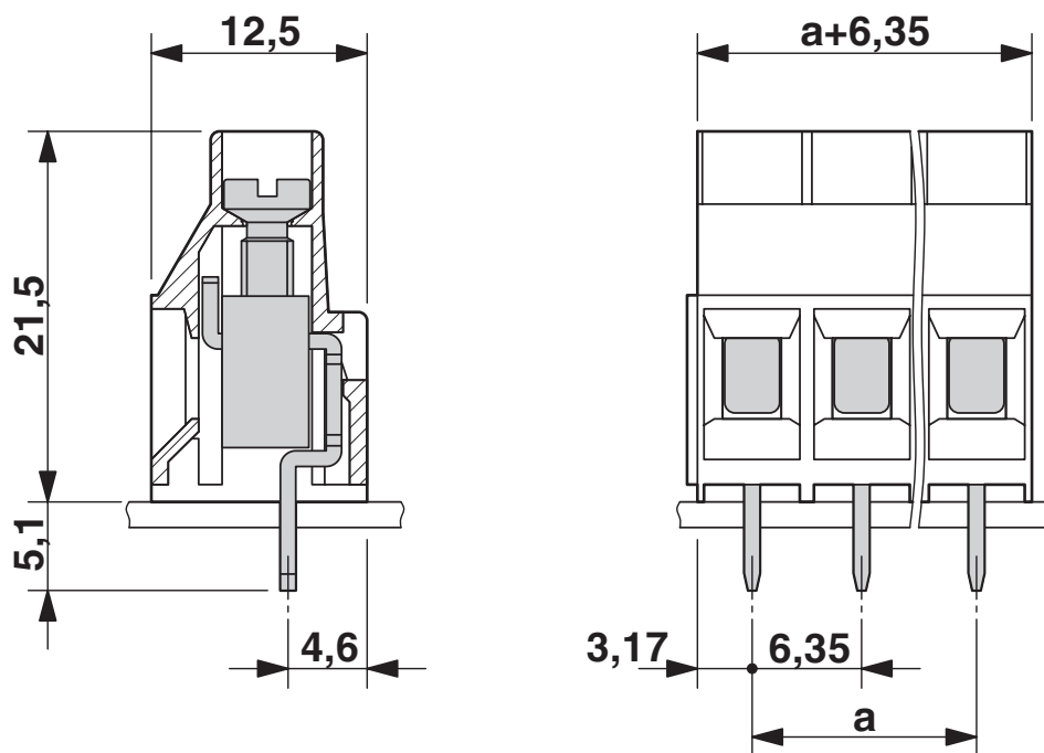
Rysunek wymiarowy
