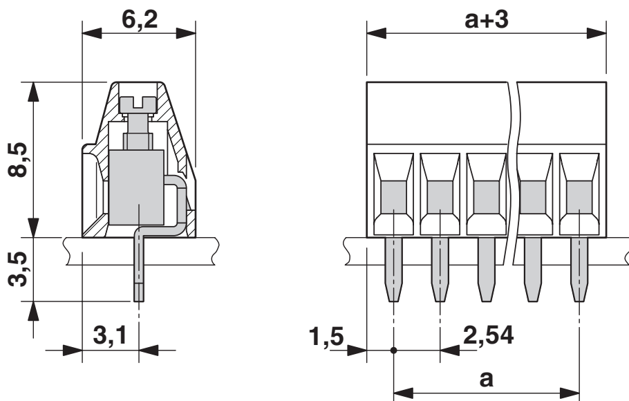
Rysunek wymiarowy
