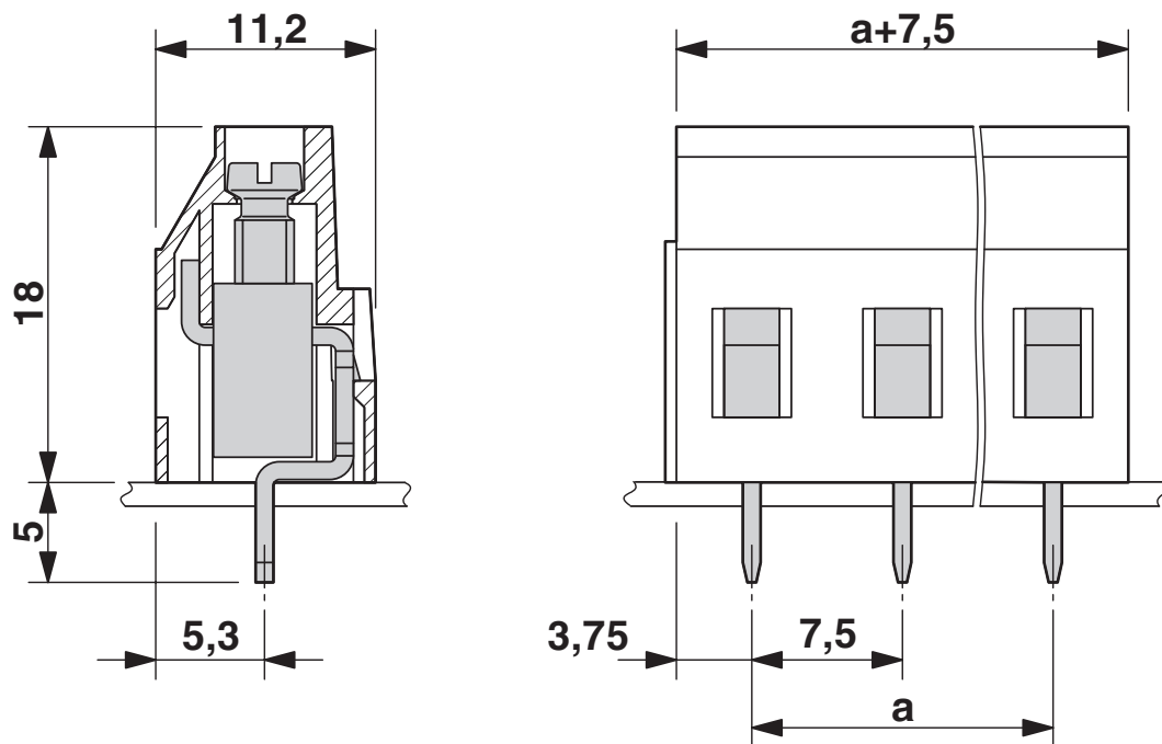
Rysunek wymiarowy
