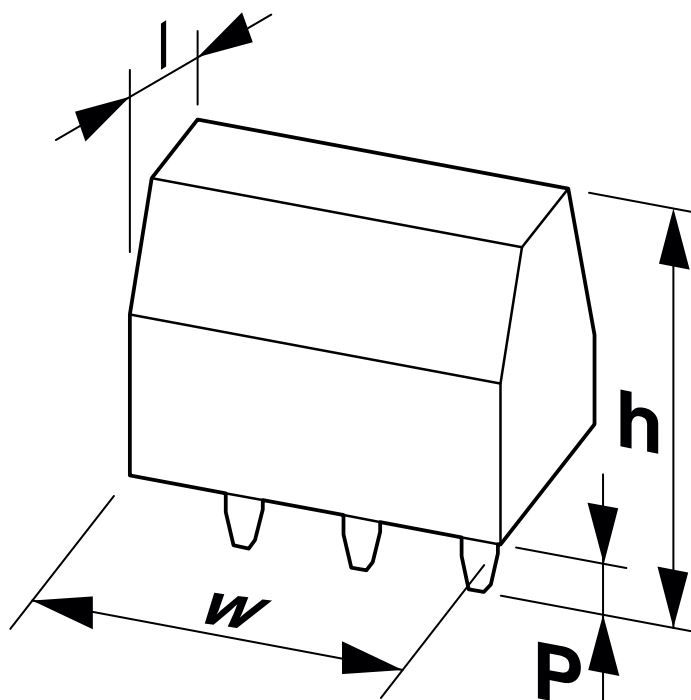
Rysunek wymiarowy
