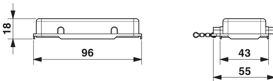
Rysunek wymiarowy
