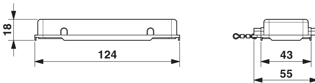
Rysunek wymiarowy
