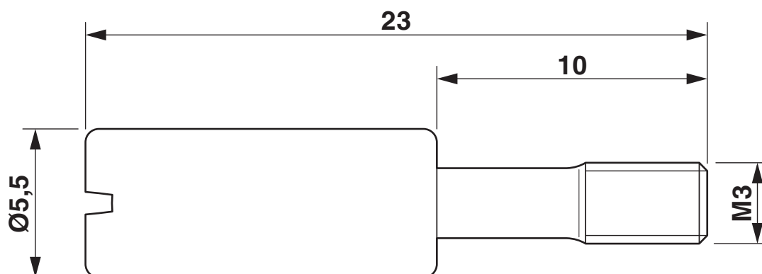
Rysunek wymiarowy
