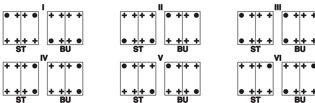
Kodowanie obudów z dwiema wkładkami stykowymi
