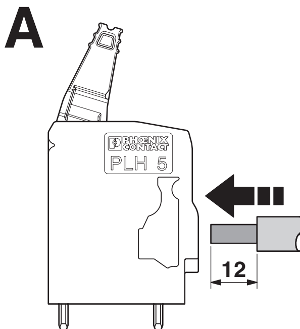
rysunek funkcyjny
