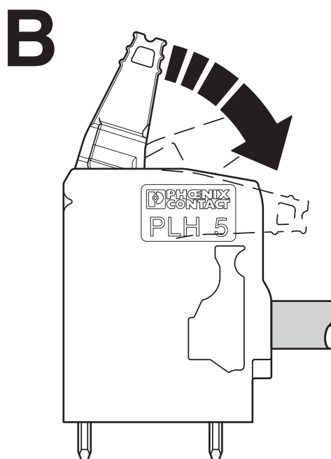
rysunek funkcyjny
