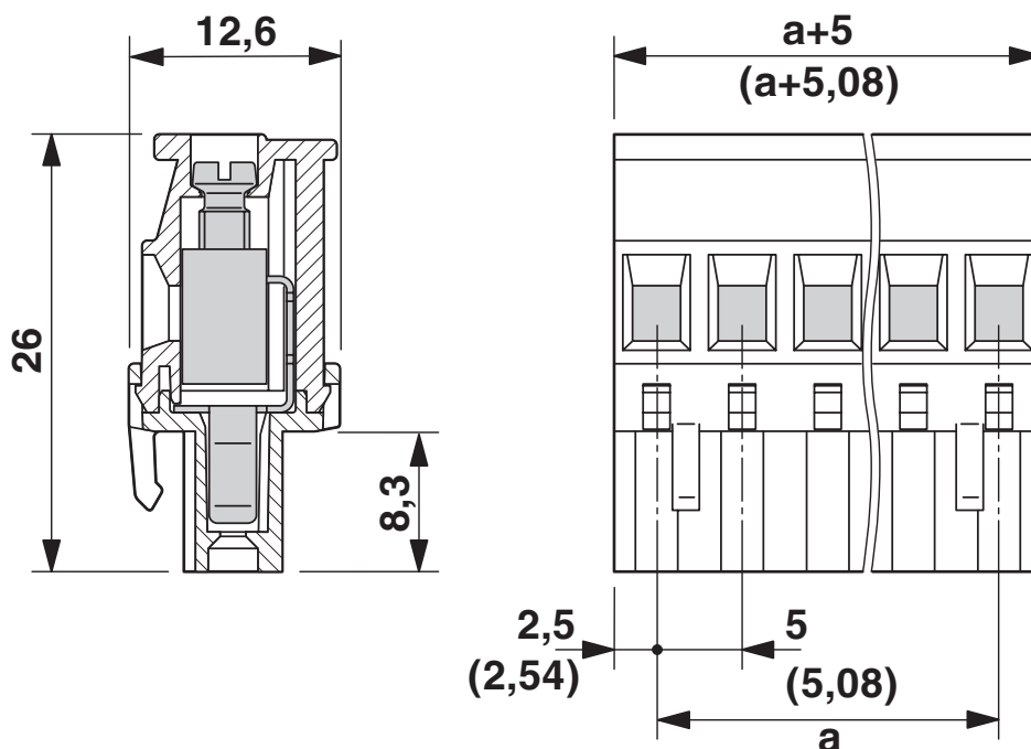
Rysunek wymiarowy
