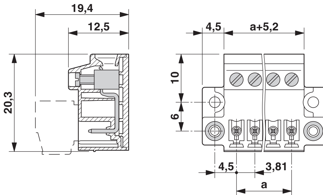
Rysunek wymiarowy
