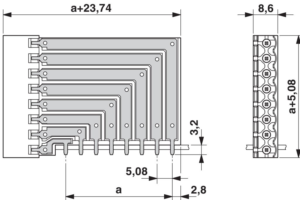
Rysunek wymiarowy
