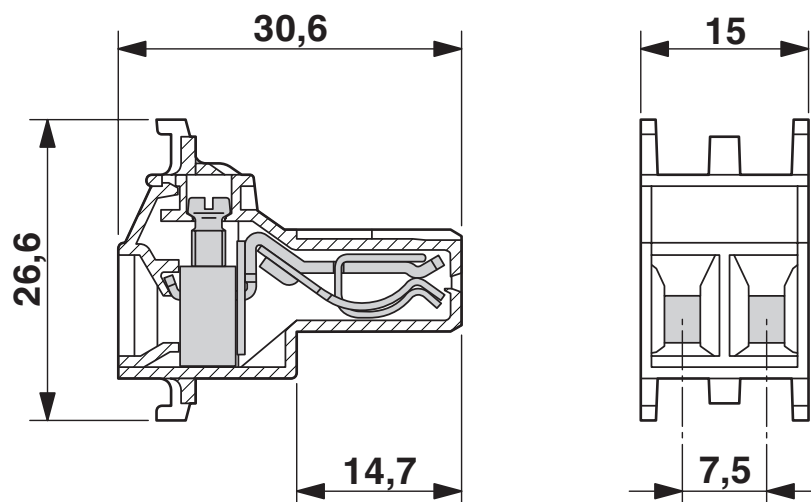
Rysunek wymiarowy
