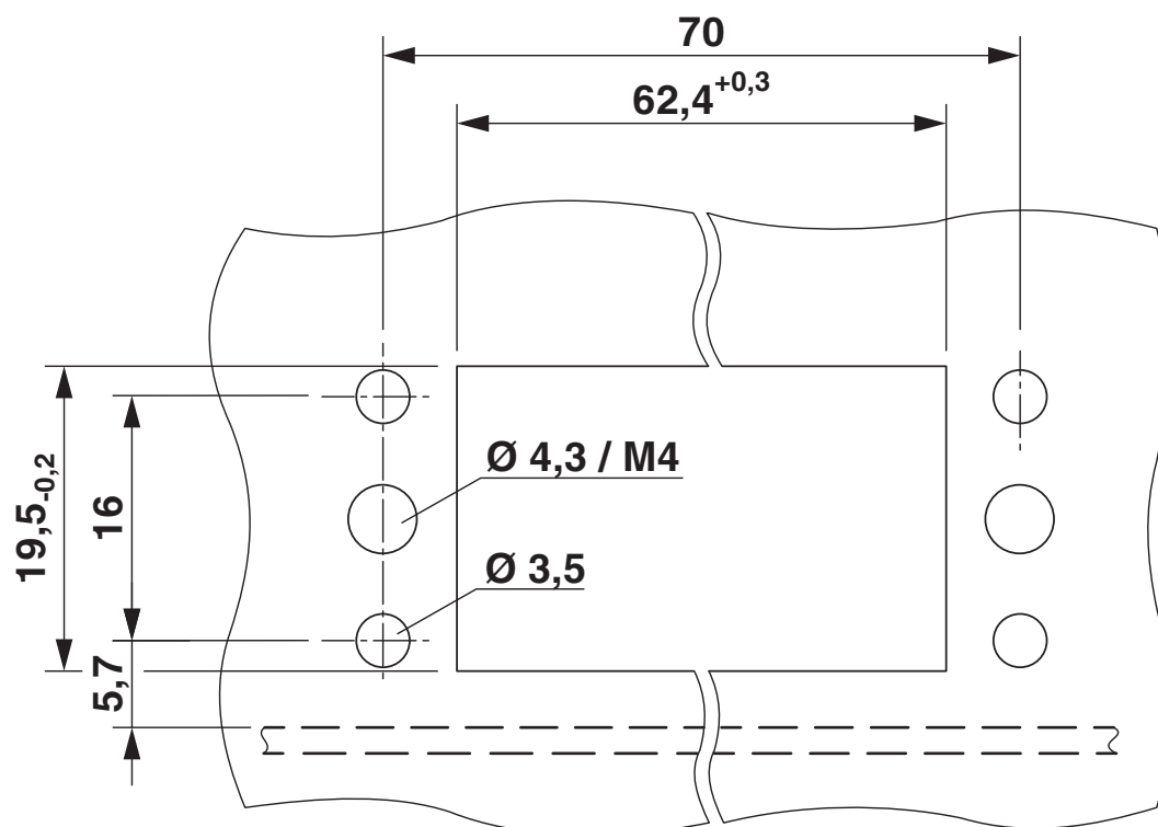
Rysunek wymiarowy
