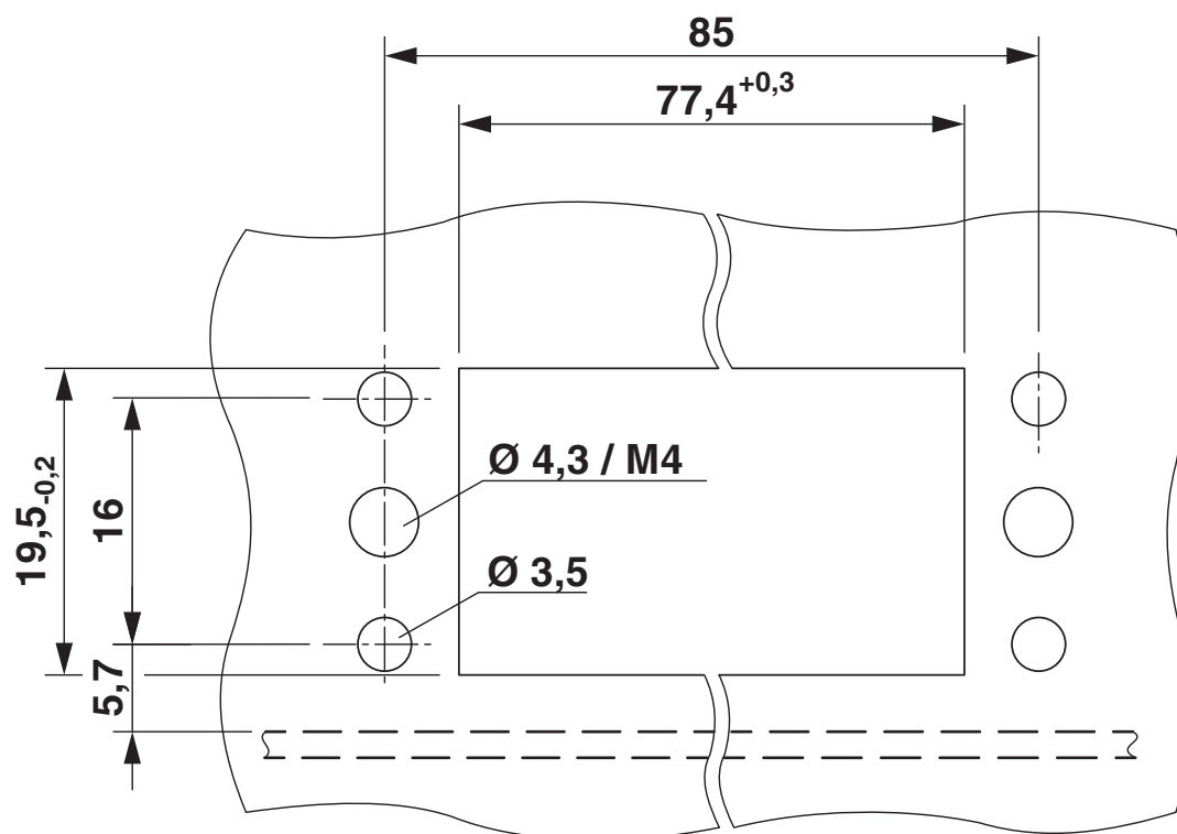
Rysunek wymiarowy
