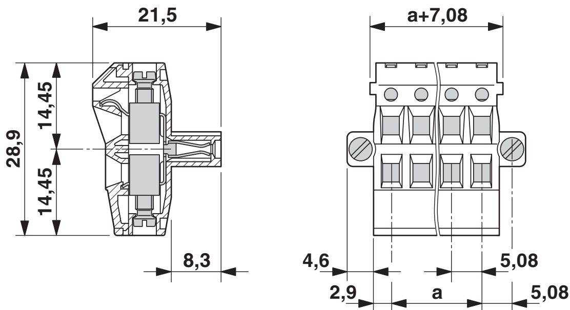
Rysunek wymiarowy
