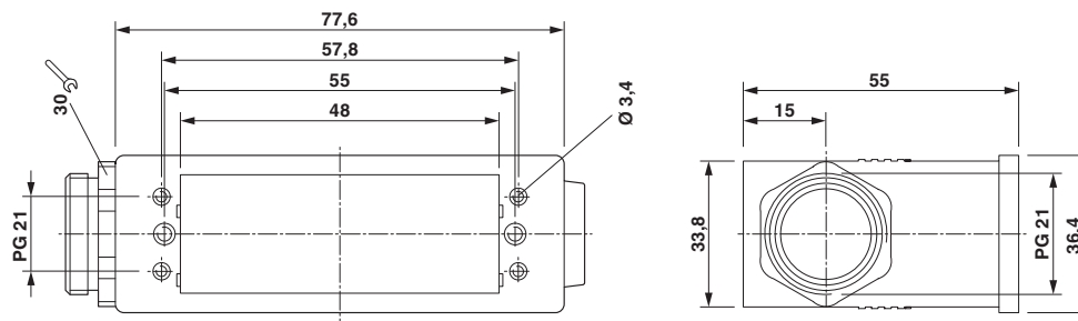
Rysunek wymiarowy
