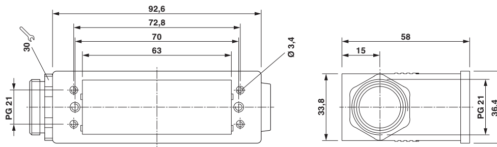
Rysunek wymiarowy
