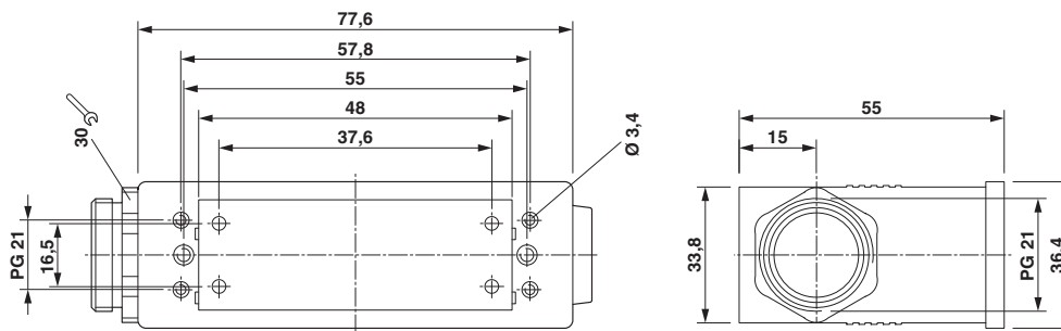
Rysunek wymiarowy
