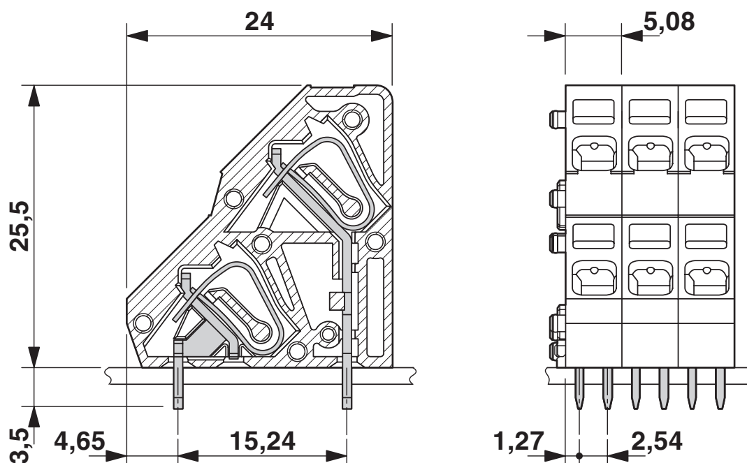
Rysunek wymiarowy
