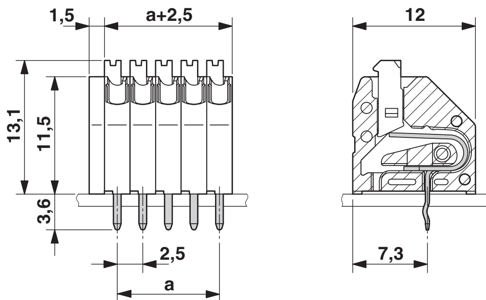
Rysunek wymiarowy
