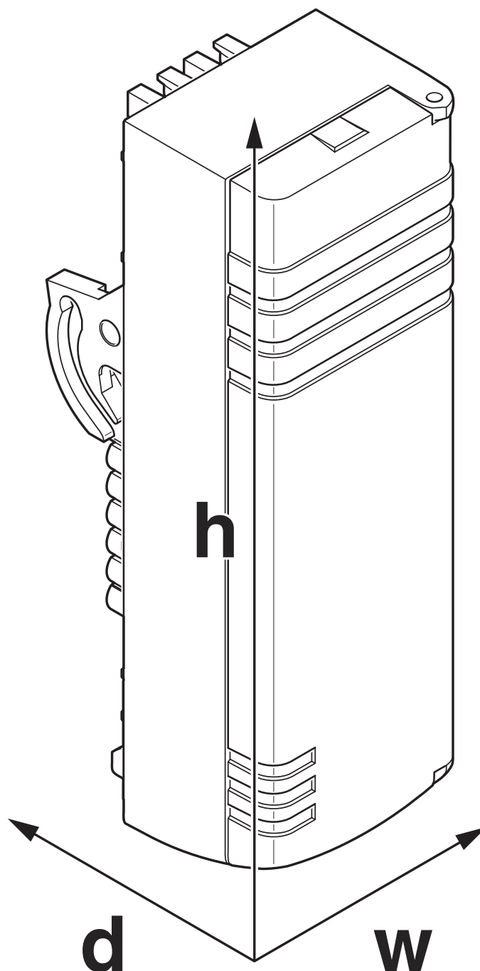
Rysunek wymiarowy
