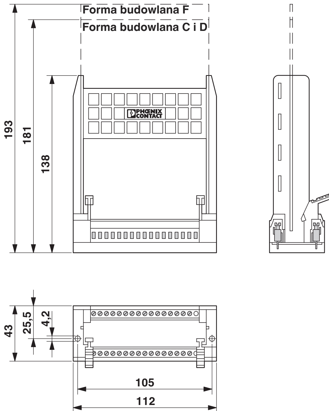
Rysunek wymiarowy
