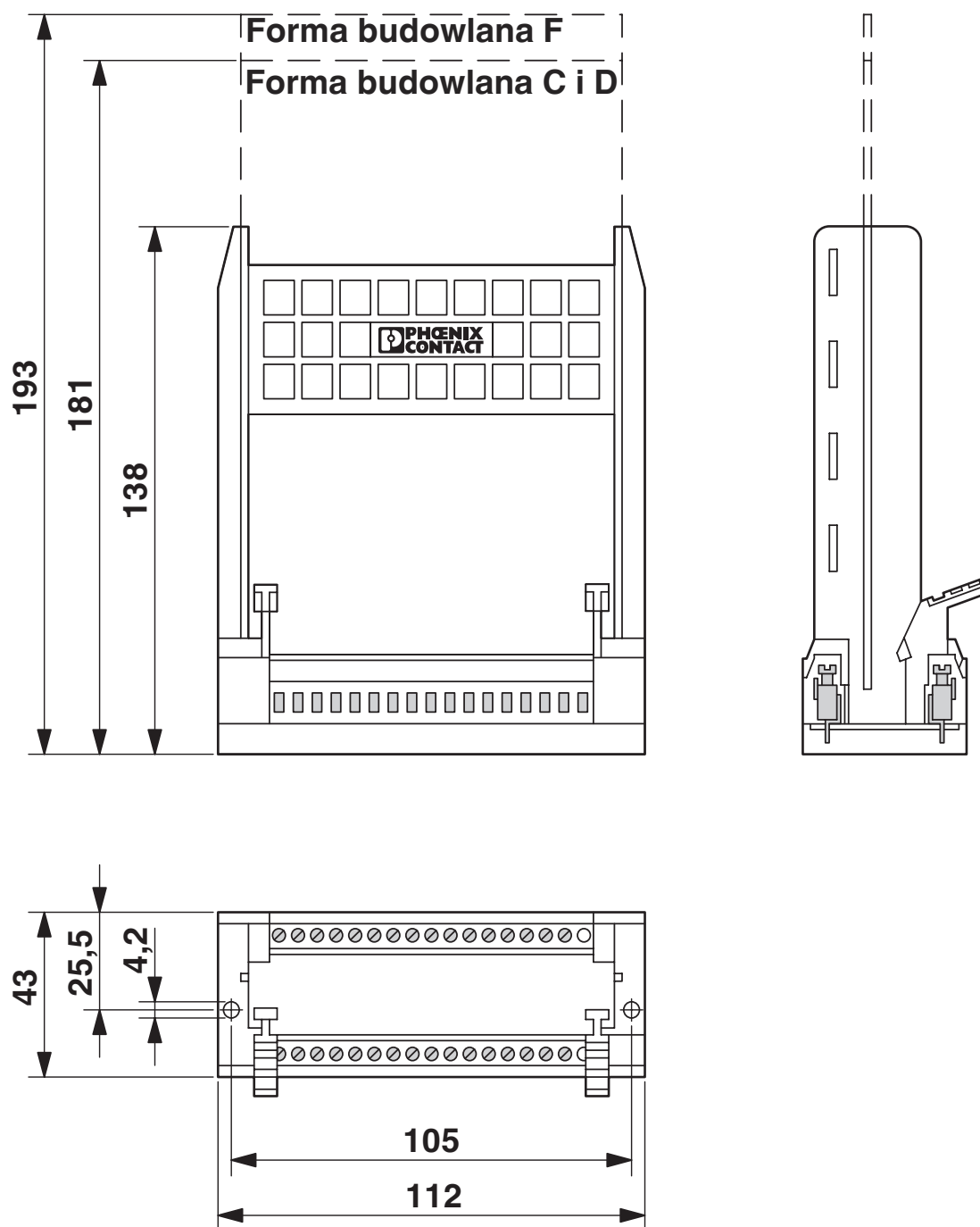
Rysunek wymiarowy
