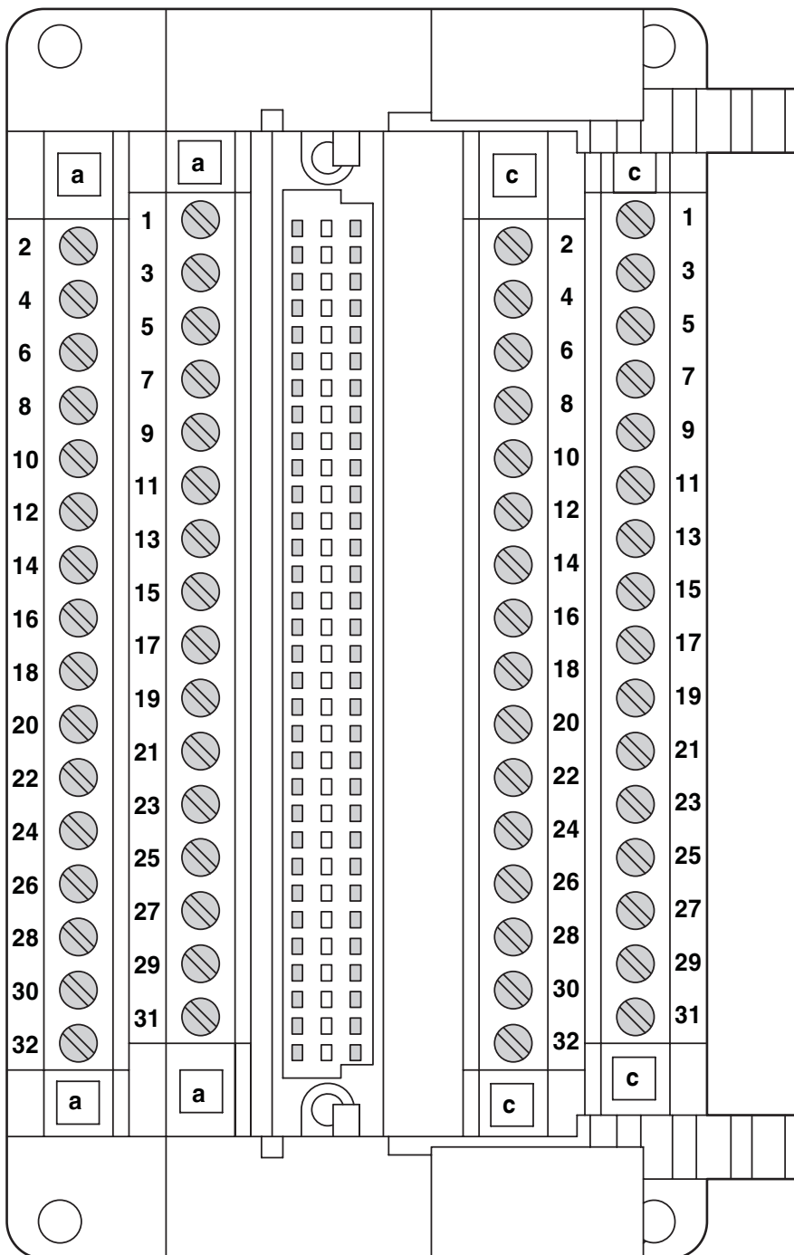
Rysunek schematyczny
