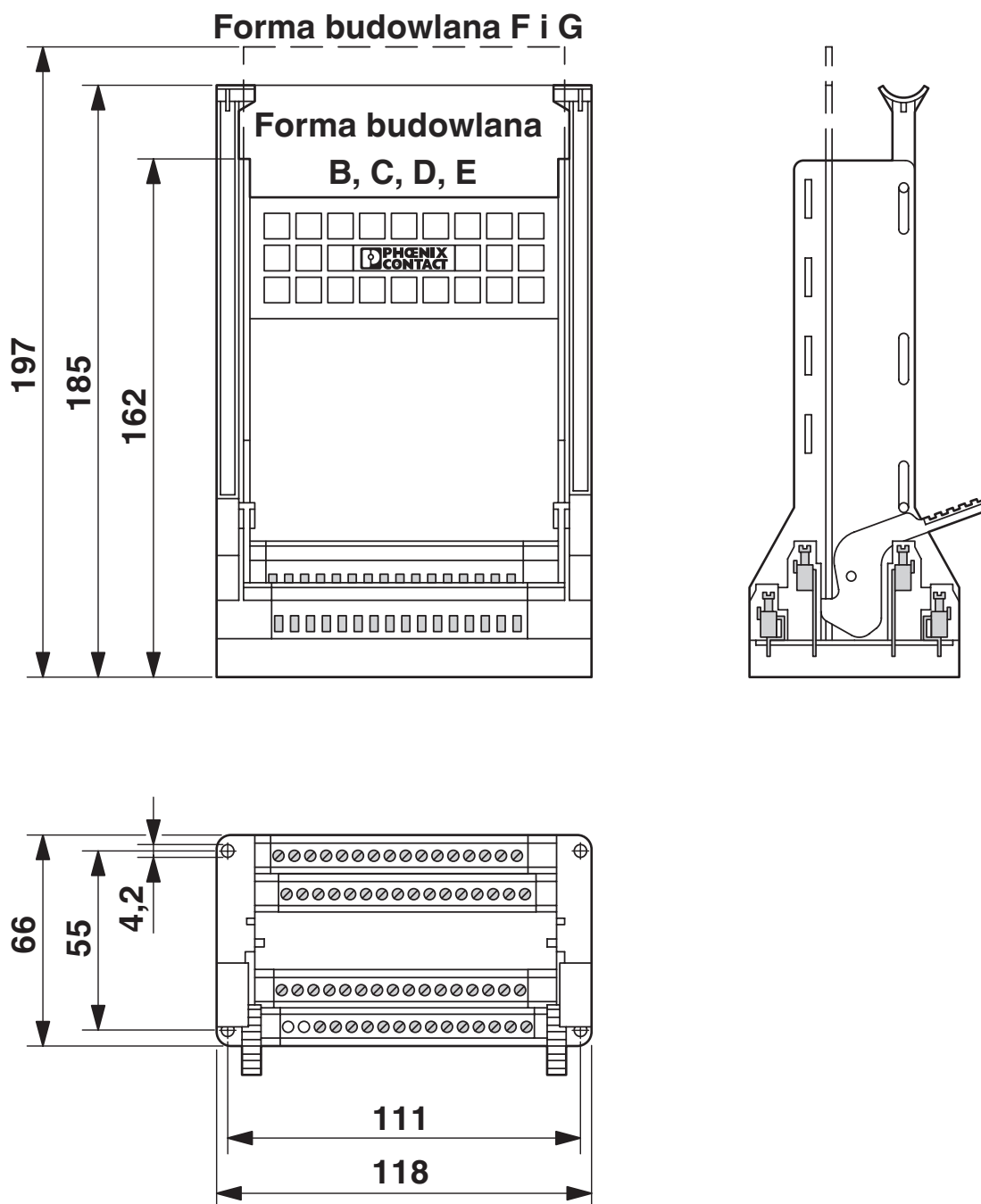
Rysunek wymiarowy
