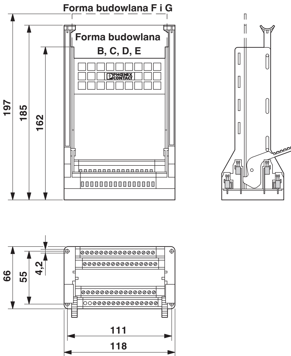
Rysunek wymiarowy
