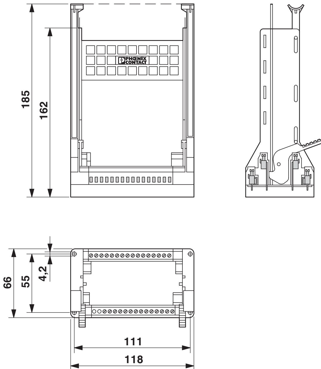
Rysunek wymiarowy
