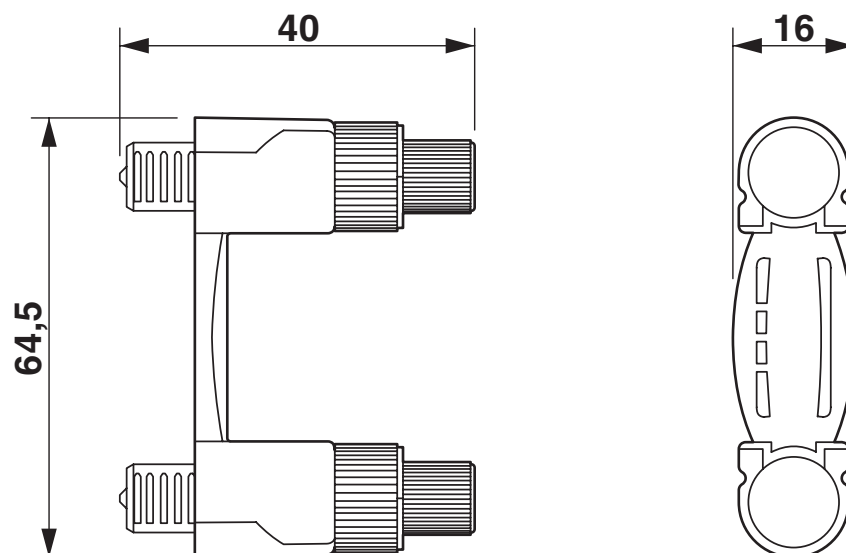
Rysunek wymiarowy
