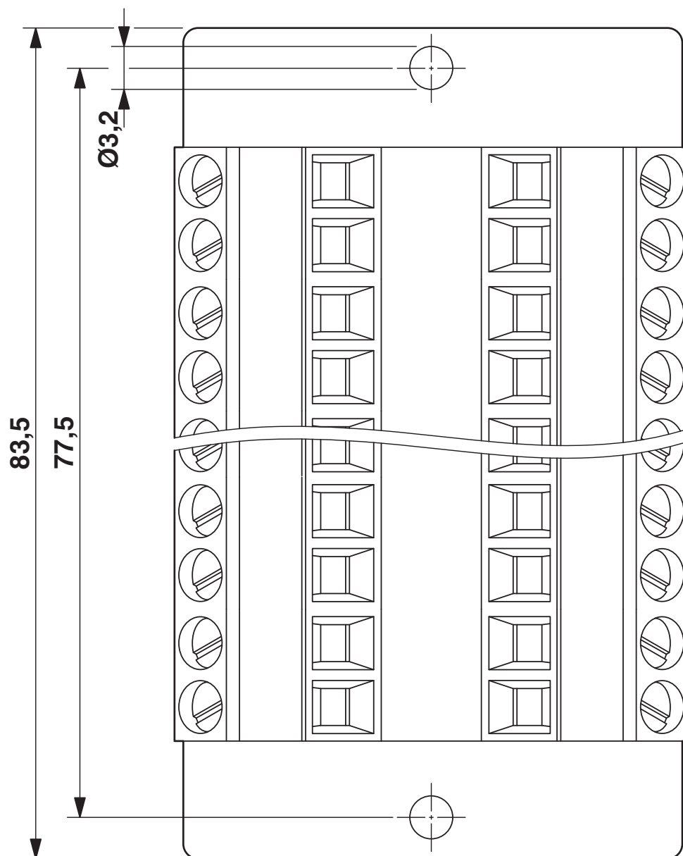
Rysunek wymiarowy
