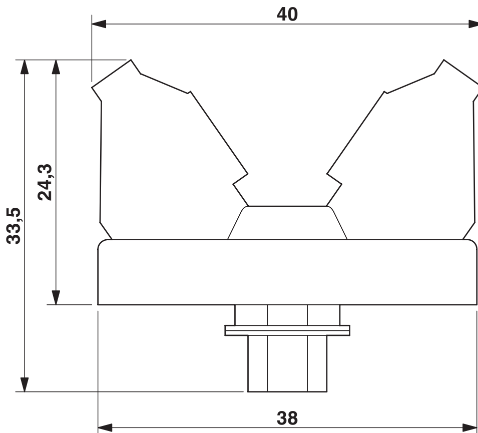
Rysunek wymiarowy
