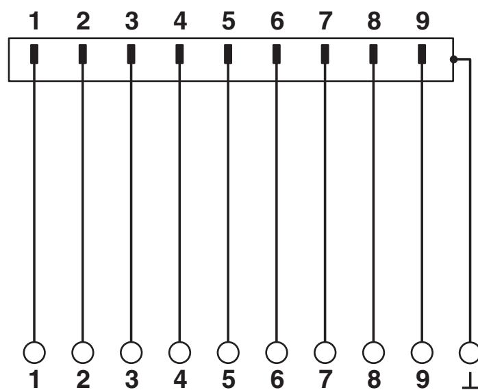
Schemat
