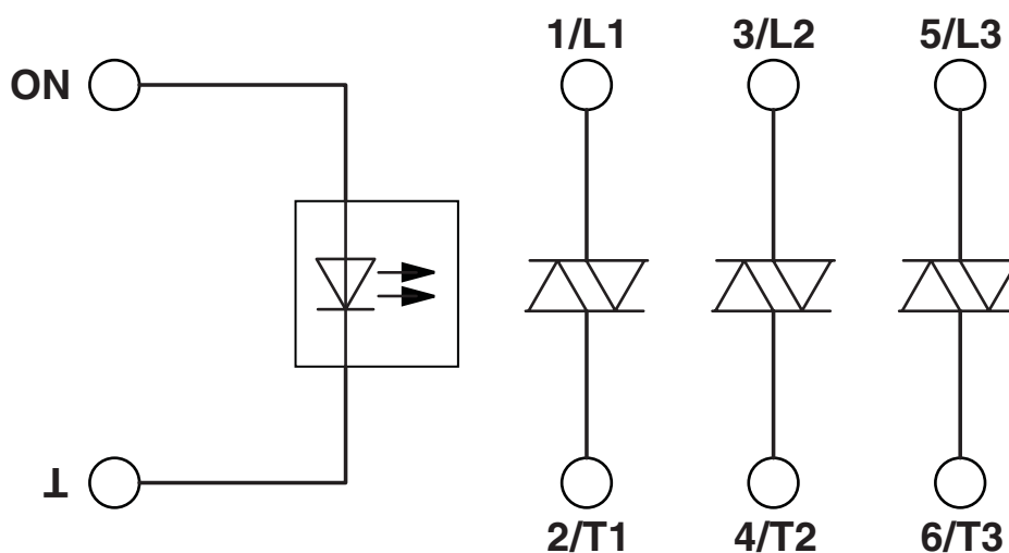
Schemat blokowy
