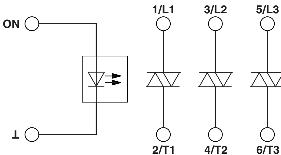
Schemat blokowy
