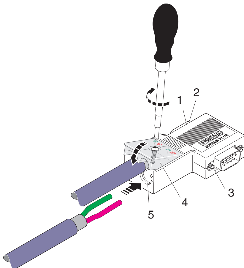
Rysunek schematyczny
