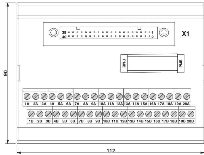
Rysunek wymiarowy
