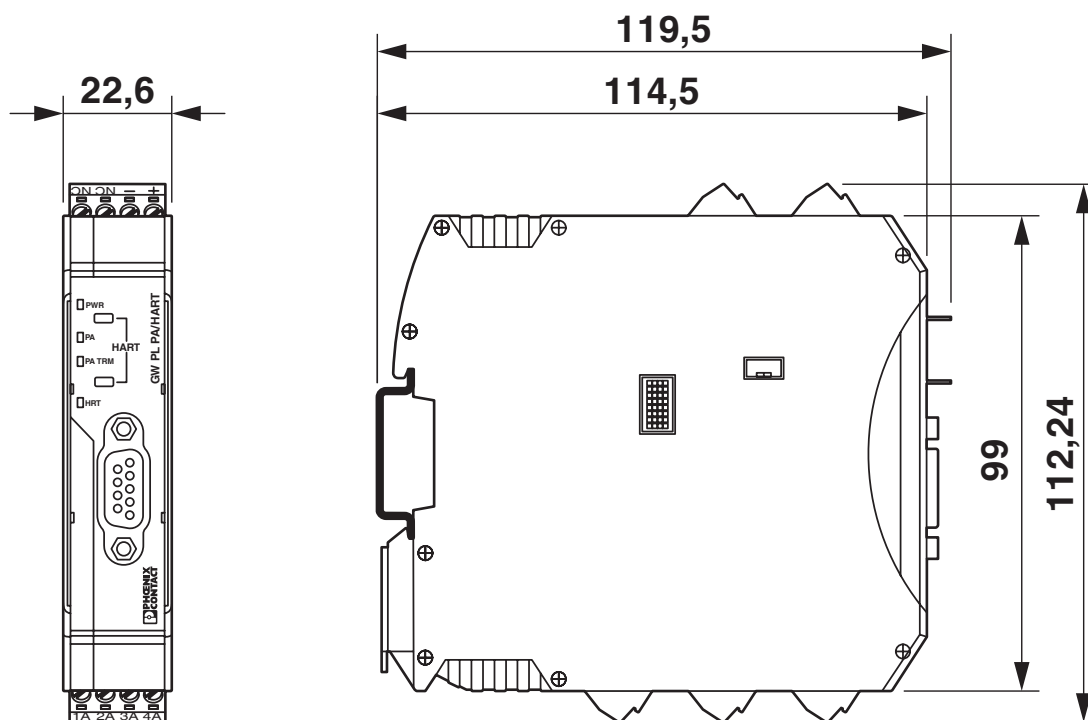
Rysunek wymiarowy
