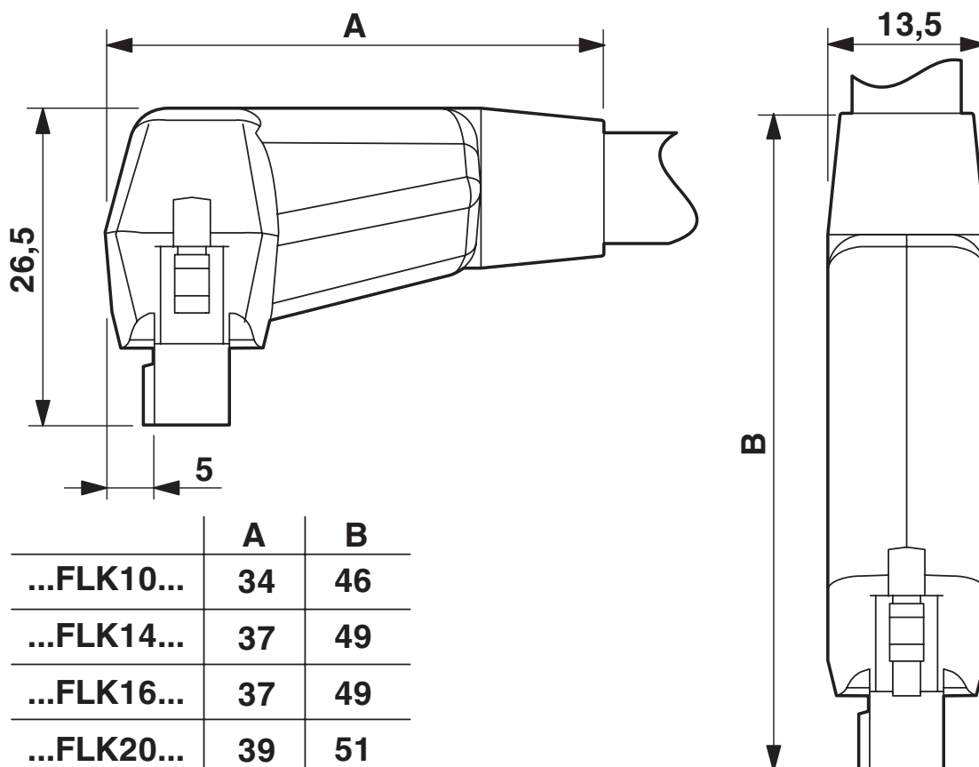
Rysunek wymiarowy
