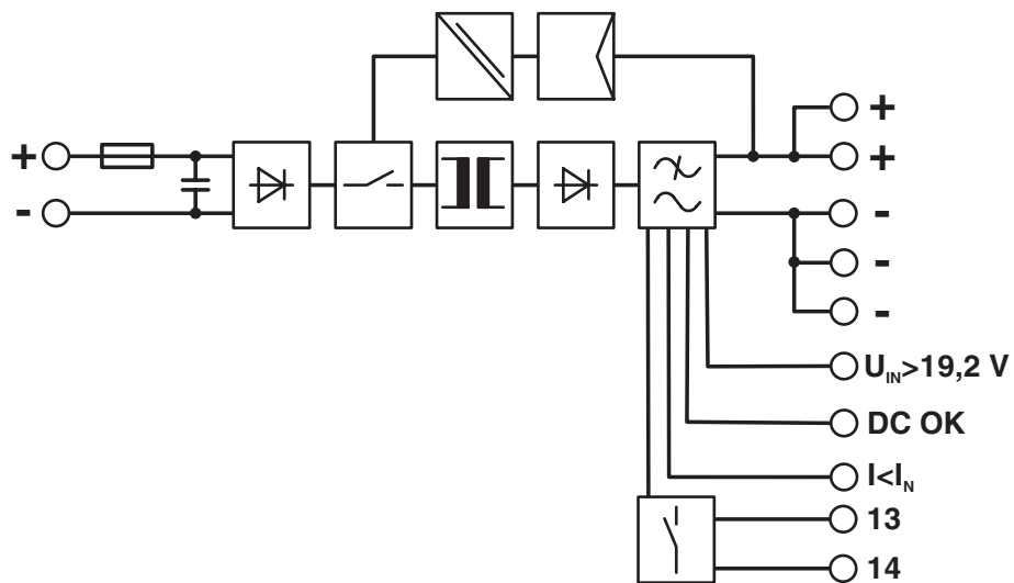
Schemat blokowy
